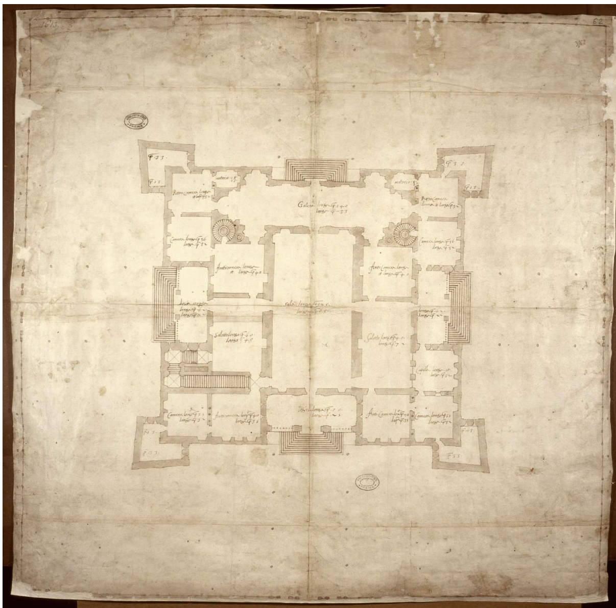
Figura 9. Francesco Paciotta, progetto per il palazzo Farnese di Piacenza, disegno su carta, seconda metà XVI secolo. Parma, Archivio Storico di Parma, Mappe e disegni, vol. 3, n. 62 (su concessione del Ministero della Cultura).
