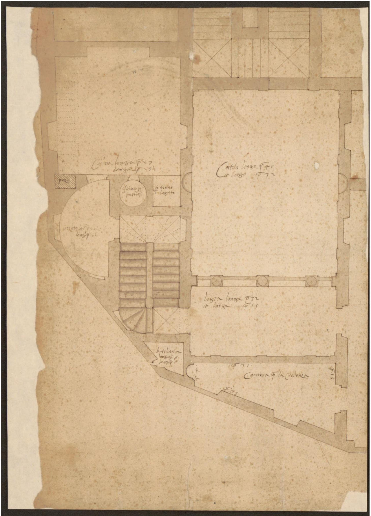
Figura 8. Francesco Paciotta (attr.), Progetto per il retro di Palazzo Torres-Lancellotti, disegno su carta, 1548-1550 circa. Roma, Archivio Storico di Roma, Ospedale di San Giacomo degli Incurabili, b. 1505, 1/92 (su concessione del Ministero della Cultura).
