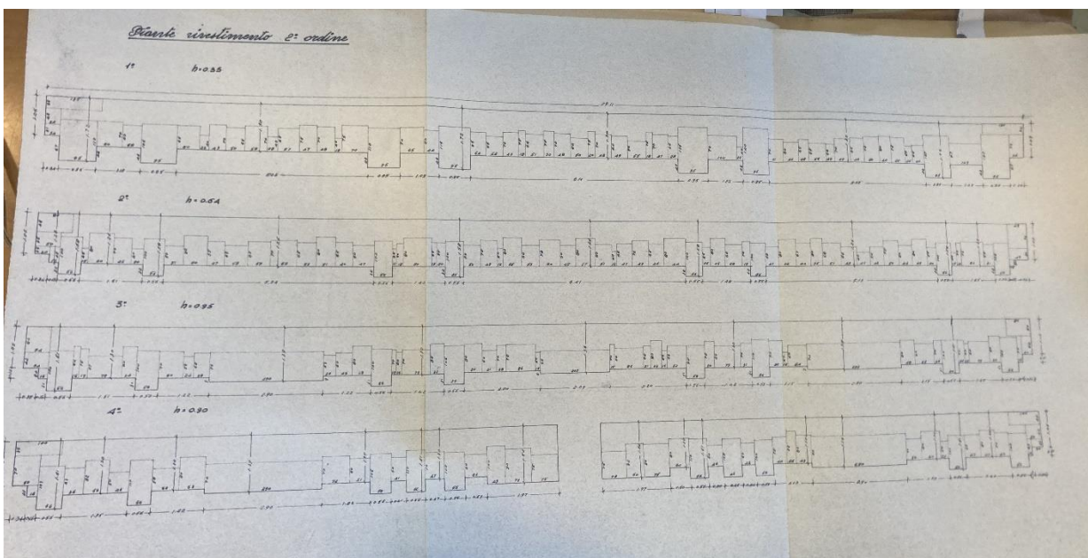
9. Uno stralcio delle "piante rivestimento" con la misurazione della profondità dei conci della facciata, sezionata a diverse altezze su entrambi i livelli smontati (AS-Aq, Genio Civile, busta 18).
