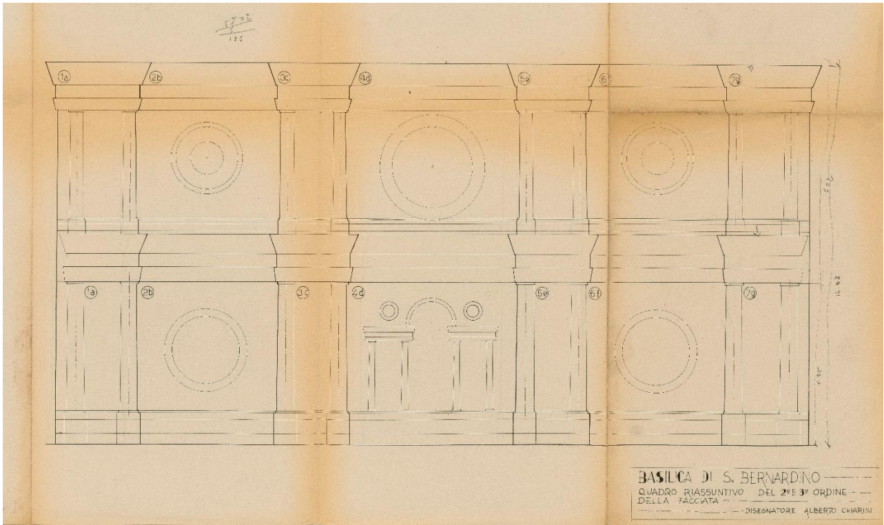
6. Il disegno d'insieme (relativo ai due ordini superiori della facciata) con l'individuazione delle porzioni smontate (AS-Aq).
